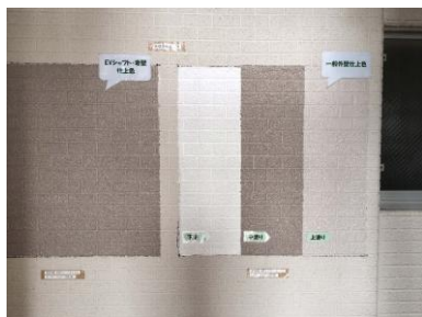
④ 外壁：下塗り・中塗り・上塗り見本
